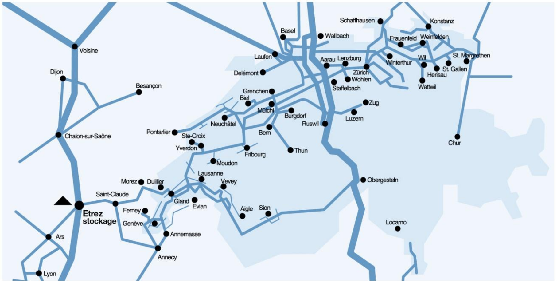
Interconnexion du réseau Gaznat au réseau européen
