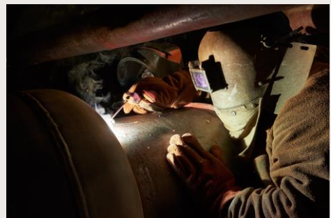
Travaux de soudure des manchons Février 2022
