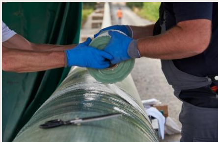
Pose du revêtement fibre de verre Août 2021
